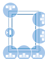
Allseitiger Beschlag mit Achtkantverschlussbolzen + Sicherheitsschließblechen
